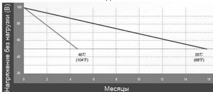
Рис. 2. ГРАФИК ЗАВИСИМОСТИ САМОРАЗРЯДА БАТАРЕИ ОТ ТЕМПЕРАТУРЫ
